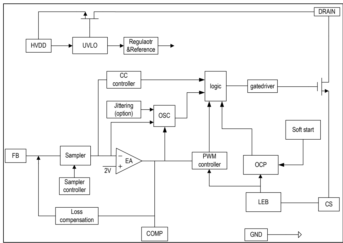
内部功能简单框图
